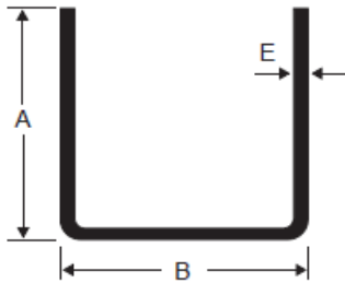
Dimensiones Dimensions / Dimensions AxBxAxE mm
